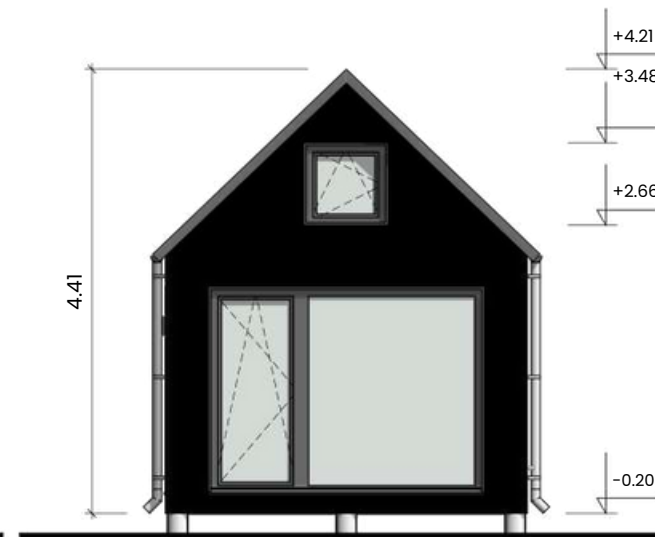
F2 FASADAS 1:75
