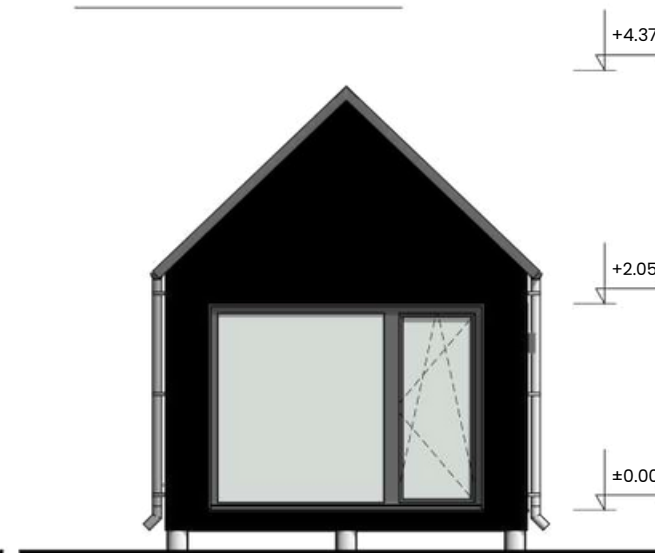
F4 FASĀDE 1:75
